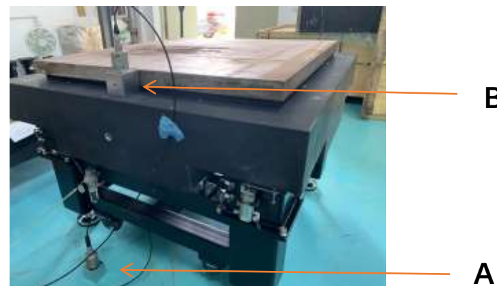
图2 检测现场
