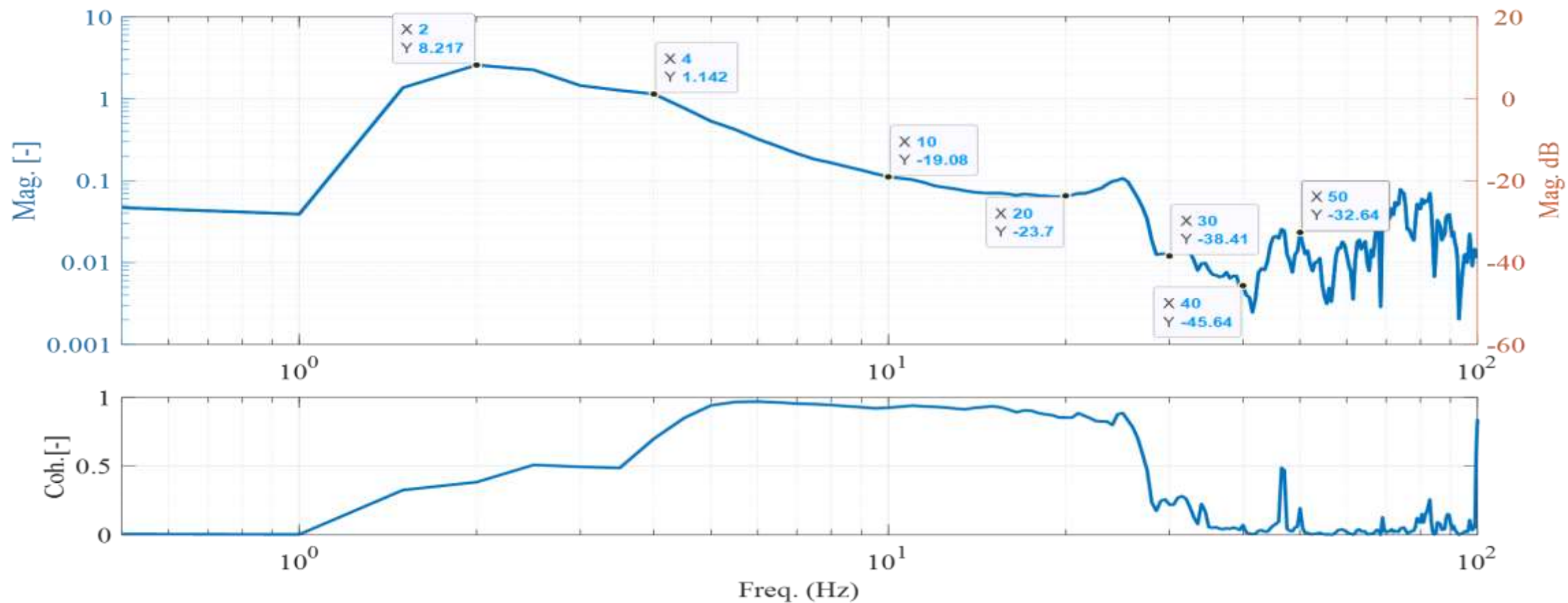
图5 传递率
